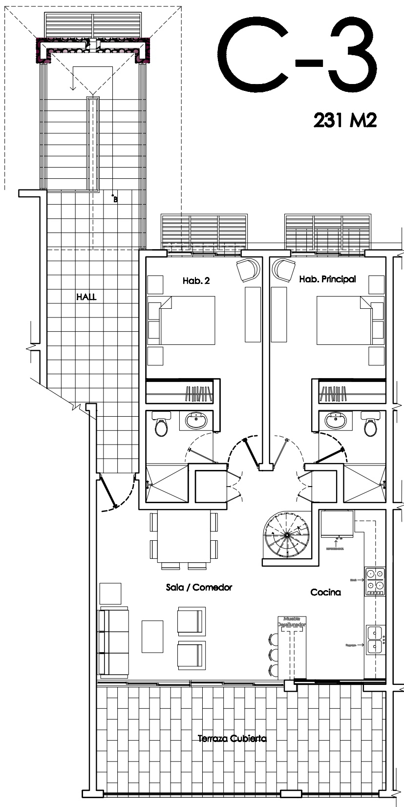
Planta Arq. 3er. Nivel Bloque central este
