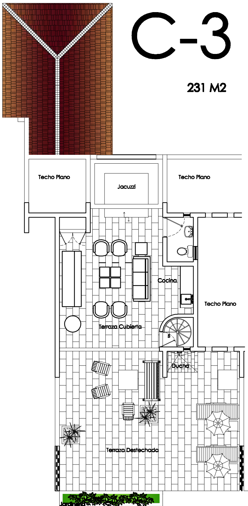
Planta Arq. 4to. Nivel Bloque Central este
